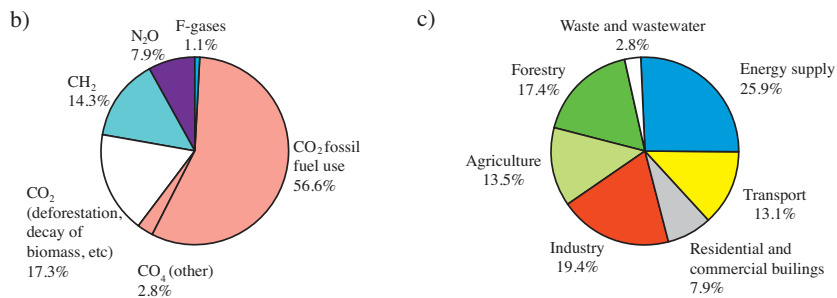
Figur b) Andel af forskellige CO 2 -ækvivalenter i den samlede globale udledning i 2004. (kilde: IPCC)
